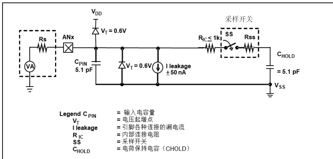
图 21: 模拟输入模型
