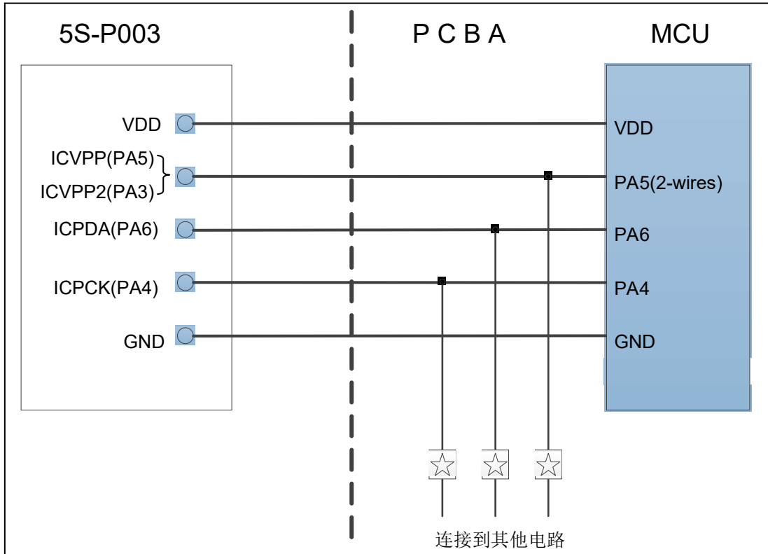
图 23：在板烧录原理图
