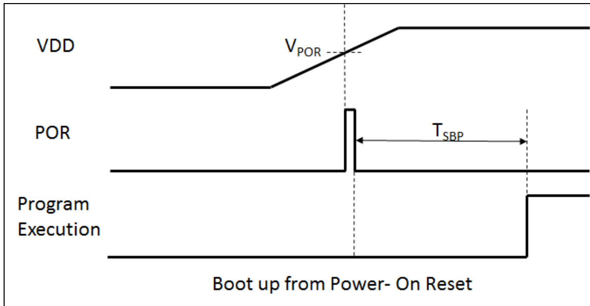
图 1：上电时序
