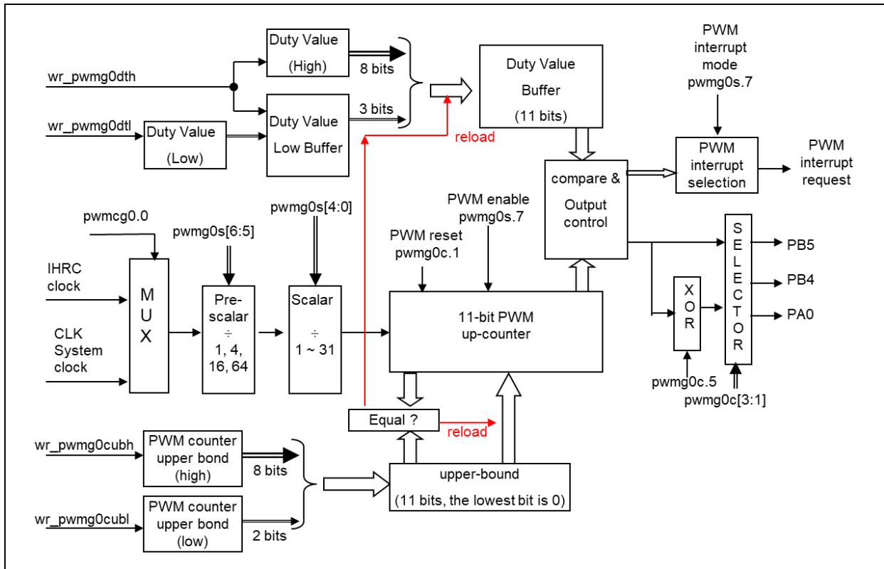
图 15: 11 位 PWM 生成器硬件框图
